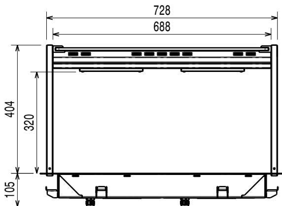
Front aanzicht
